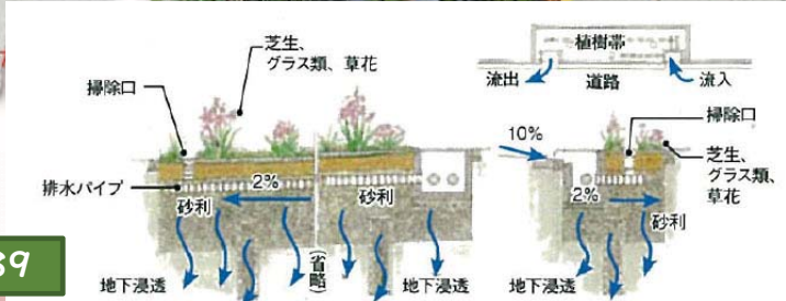
図1 道路型雨庭(上写真のタイプ)の縦断(左)、横断(右)、平面(上)のイメージ。参考文献(2)をもとに作図
